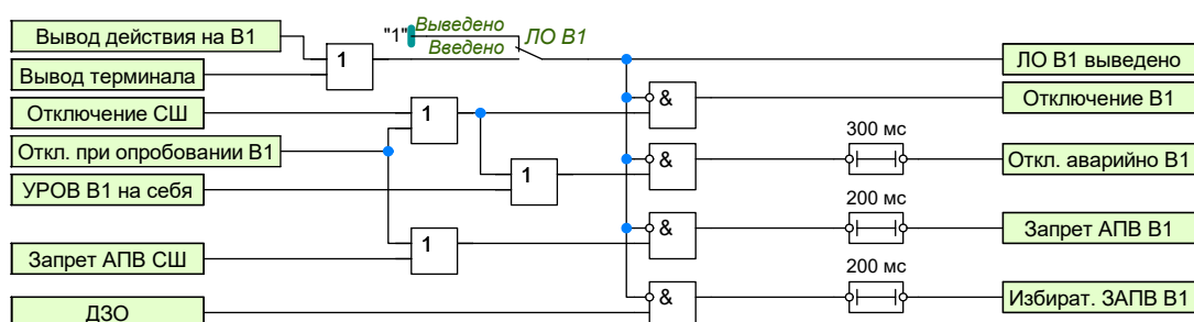
Рисунок 0.17 – Функциональный блок логики отключения первого присоединения
