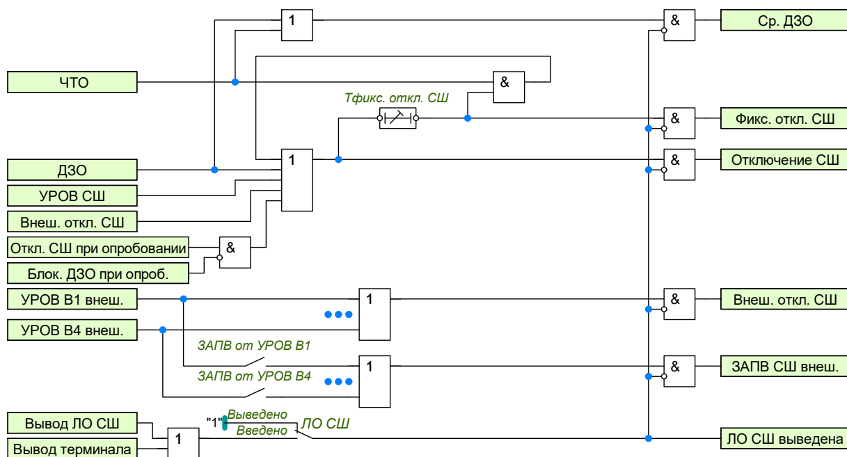
Рисунок 0.15 – Функциональный блок логики запрета АПВ
